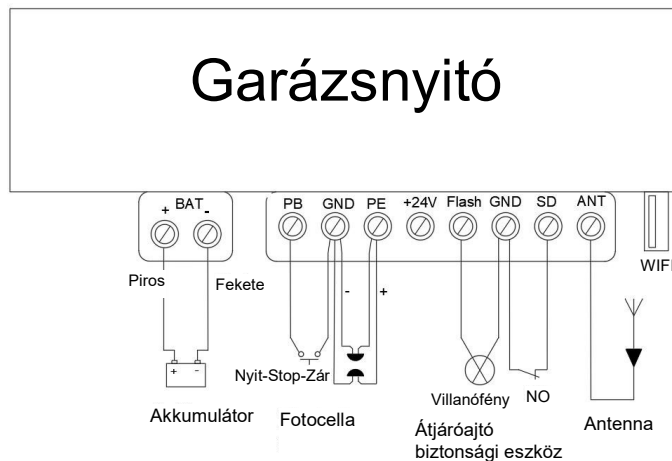
Kiegészítő terminálcsatlakozó
